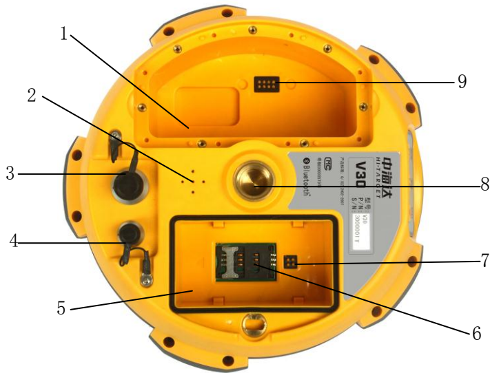
1-通信模块仓 2-喇叭 3-八芯插座及防护塞 4-五芯插座及防护塞 5-电池仓 6-SIM 卡槽 7-弹针电源座 8-连接螺孔 9-通信模块接口
